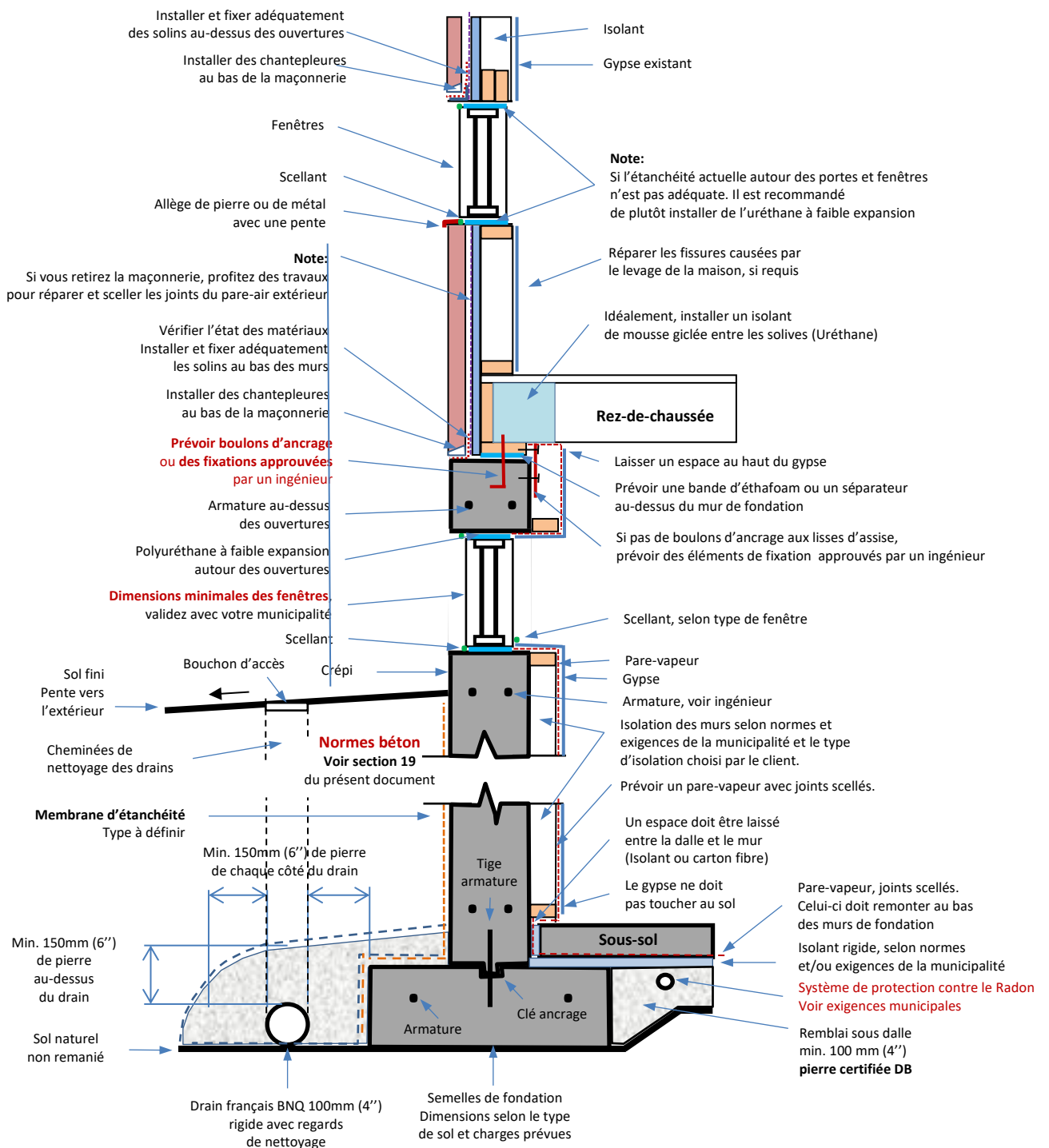
COUPE DE MUR TYPE STANDARD
