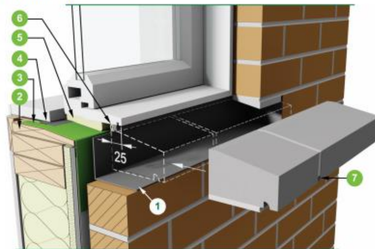
Figure 9.20.13. - 01.1 Solin métallique
