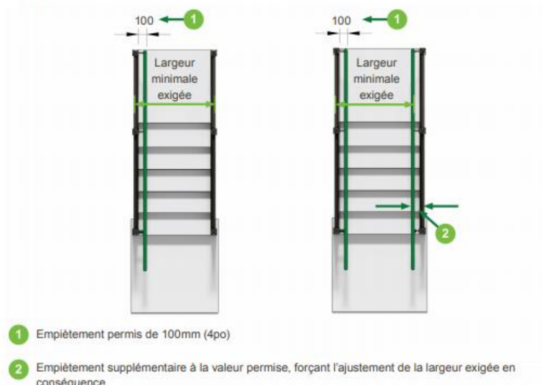
Figure 9.8.7. - 01.12 Escalier
